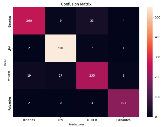
Figura 7: Matriz de confusión del testeo de un grupo de poco más de mil estrellas después de un entrenamiento Con más de cinco mil. Vemos que la predicción que más errores dió fue predecir que era una Other cuando se trataba de una binaria, y que las pulsantes y LPVs fueron muy bien predichas.
